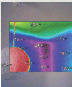
Zřetelně viditelné studené kouty místnosti v pohledu termokamery, ideální místo pro plošnou aplikaci ETERNAL In Thermo.
